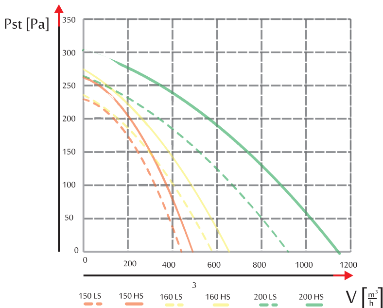
Rys. 1. Charakterystyka przepływu wydajności
